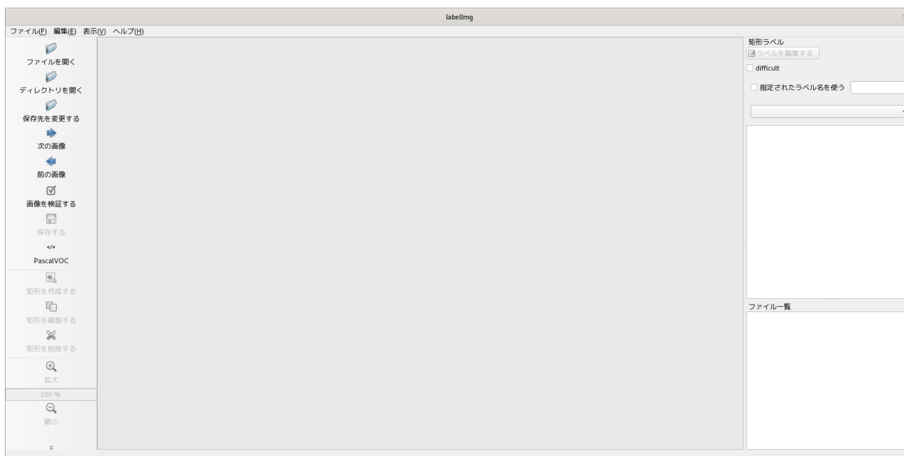
図 6.13 labellmg の起動
