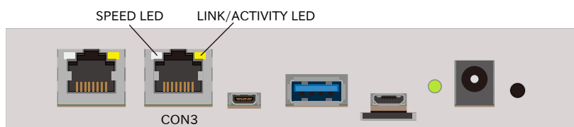
図 14.8 CON3 LAN LED 配置
