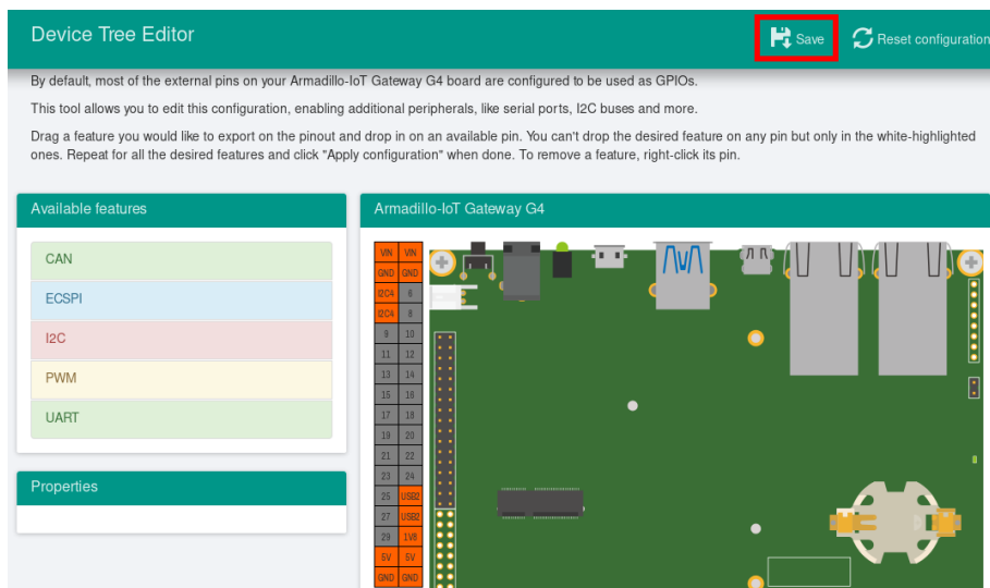
図 9.163 DTS/DTB の生成
