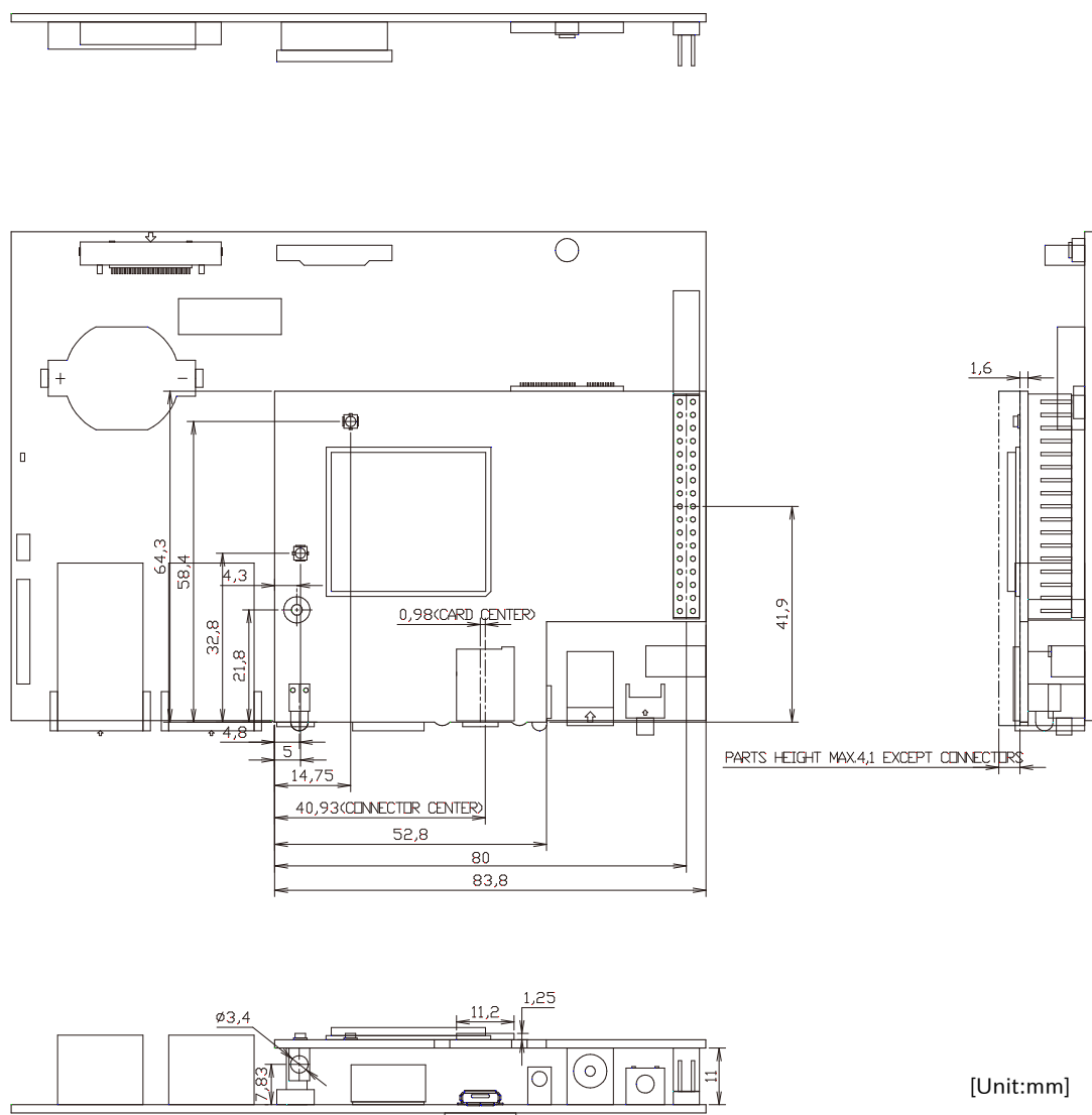
図 13.14 基板形状図(LTE モデル 追加分)
