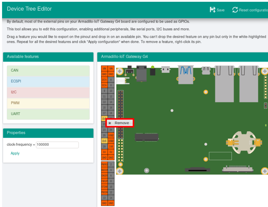
図 9.162 I2C5(SCL/SDA) の削除
