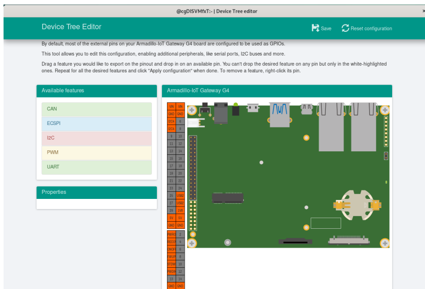
図 9.214 at-dtweb 起動画面
