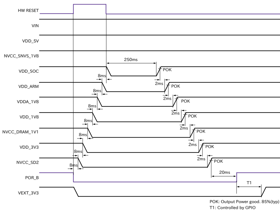
図 6.224 リセットシーケンス
