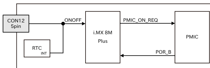
図 6.225 ONOFF 回路の構成
