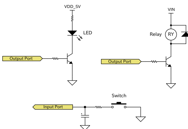
図 3.32 スイッチ、LED、リレー接続例
