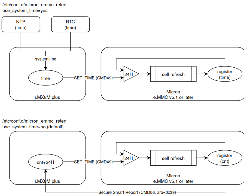
図 6.215 データリテンション開始トリガーの方式
