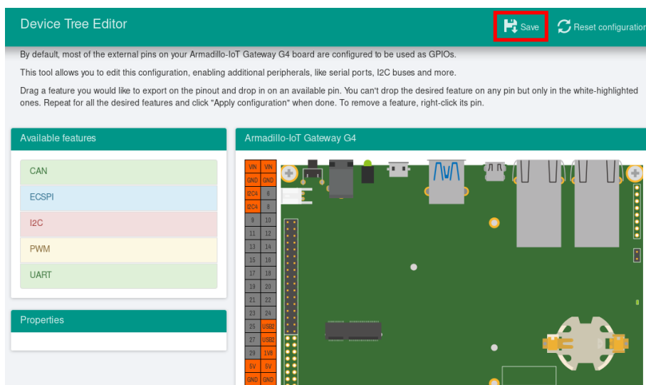
図 3.46 DTS/DTB の生成
