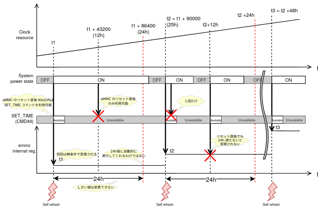
図 6.235 データリテンションの開始トリガーの動作例
