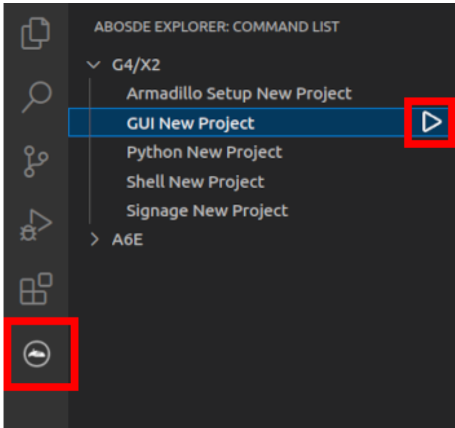
図 3.134 GUI アプリケーションのプロジェクトを作成する
