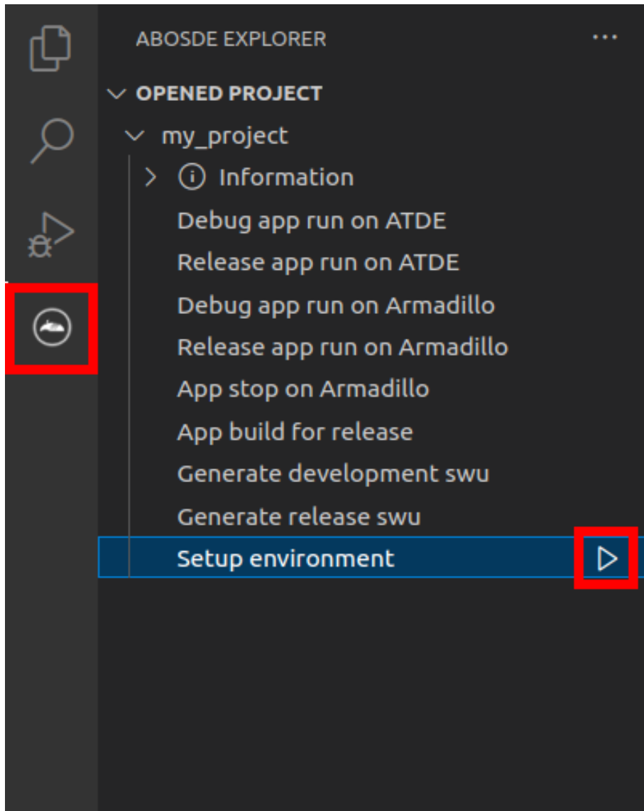
図 3.137 VSCode で初期設定を行う
