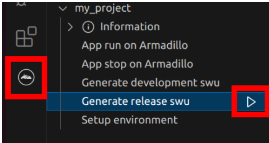
図 3.204 リリース版をビルドする
