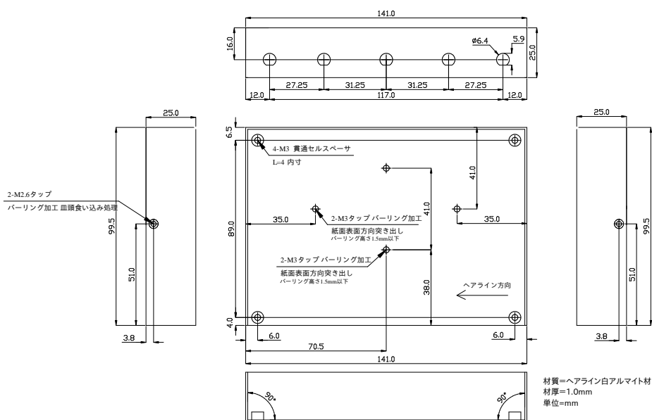
図 6.249 LTE+WLAN モデル ケース(下)形状図
