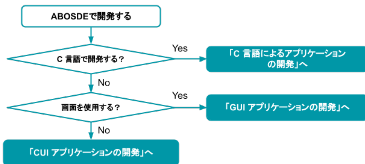
図 3.127 参照する開発手順の章を選択する流れ
