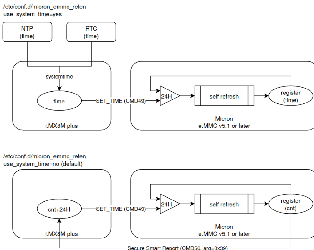
図 6.214 データリテンション開始トリガーの方式
