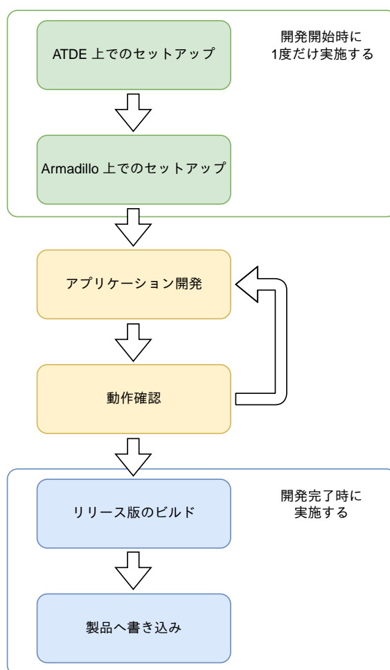
図 3.155 CUI アプリケーション開発の流れ
