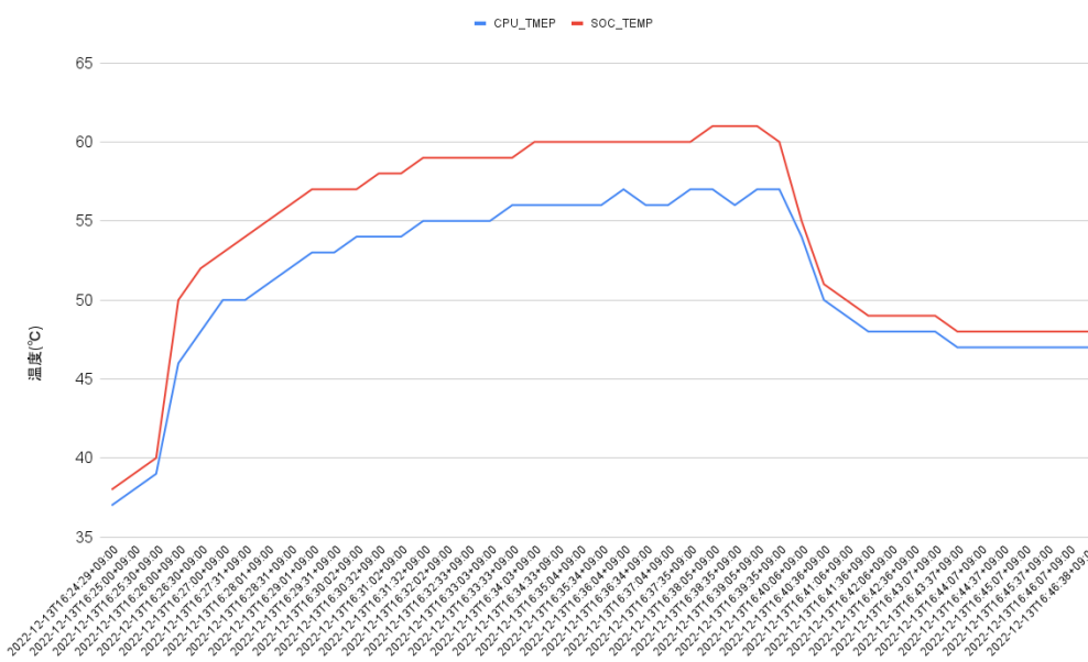
図 6.215 Armadillo-IoT ゲートウェイ G4 で取得した温度のグラフ
