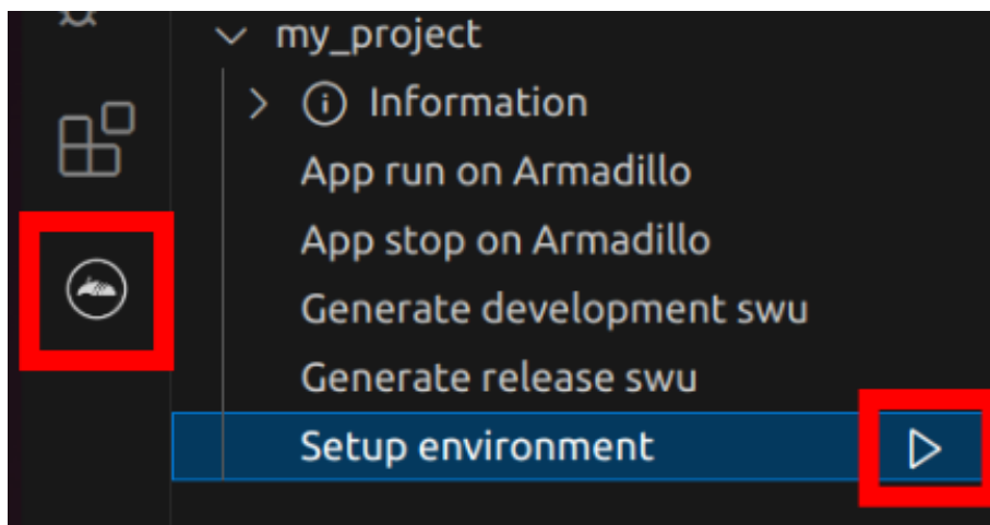
図 3.160 VSCode で初期設定を行う
