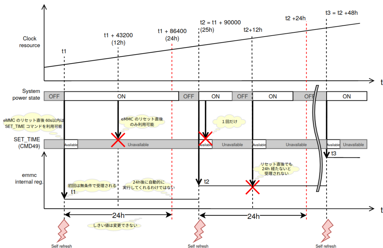
図 6.223 データリテンションの開始トリガーの動作例
