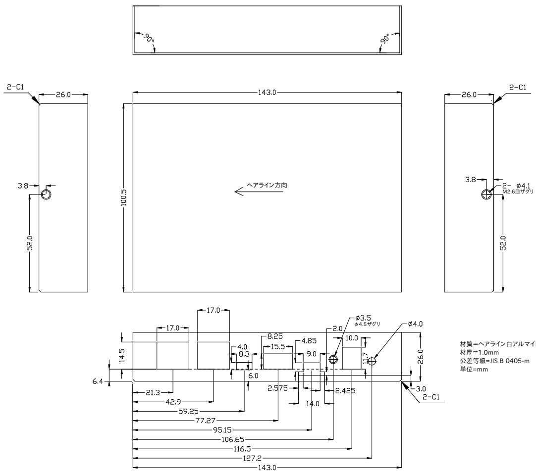
図 6.234 WLAN モデル ケース(上)形状図
