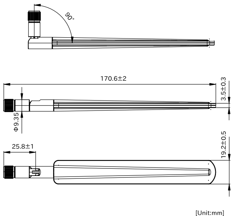
図 6.238 3G/LTE 用外付けアンテナ形状図
