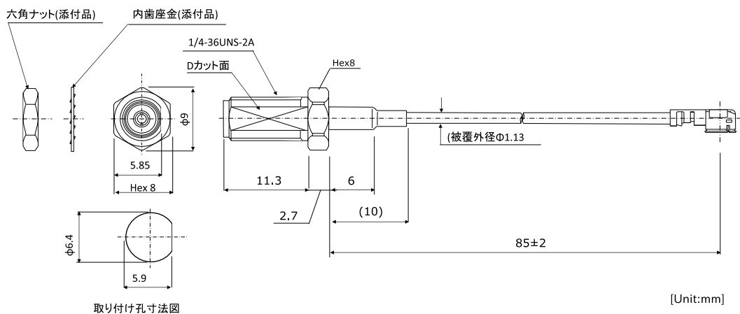
図 6.239 3G/LTE 用アンテナケーブル形状図
