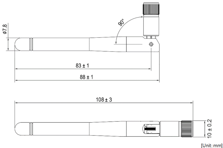
図 6.244 無線 LAN/BT 用外付けアンテナ形状図
