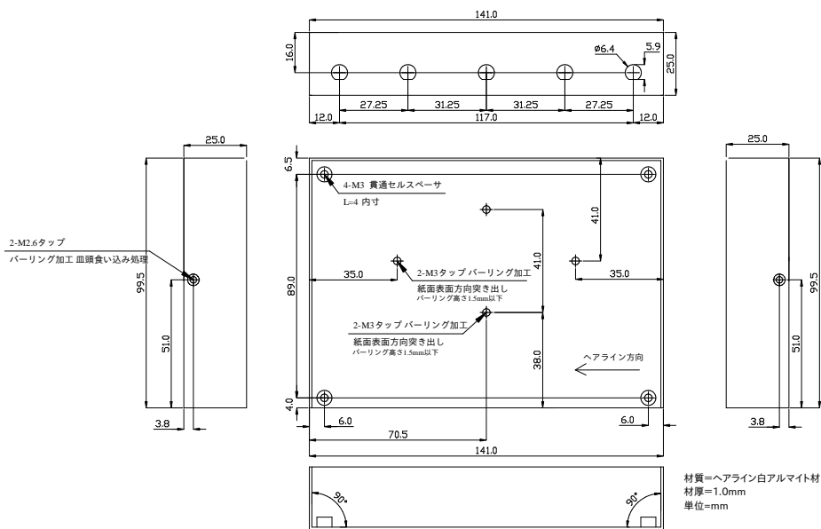
図 6.241 LTE+WLAN モデル ケース(下)形状図
