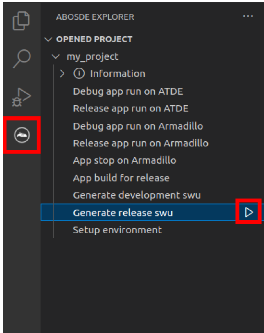
図 3.170 SWU イメージを作成する
