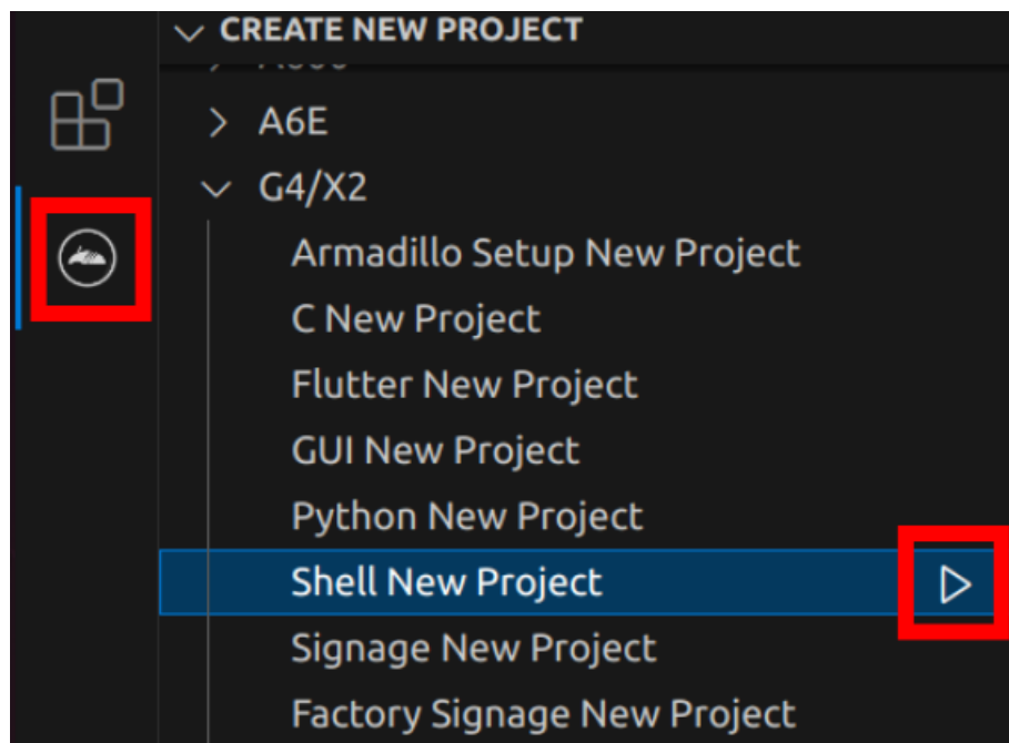
図 3.172 プロジェクトを作成する
