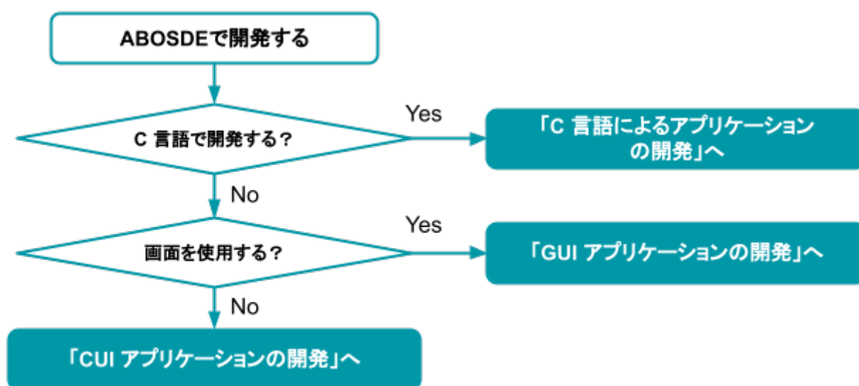
図 3.125 参照する開発手順の章を選択する流れ
