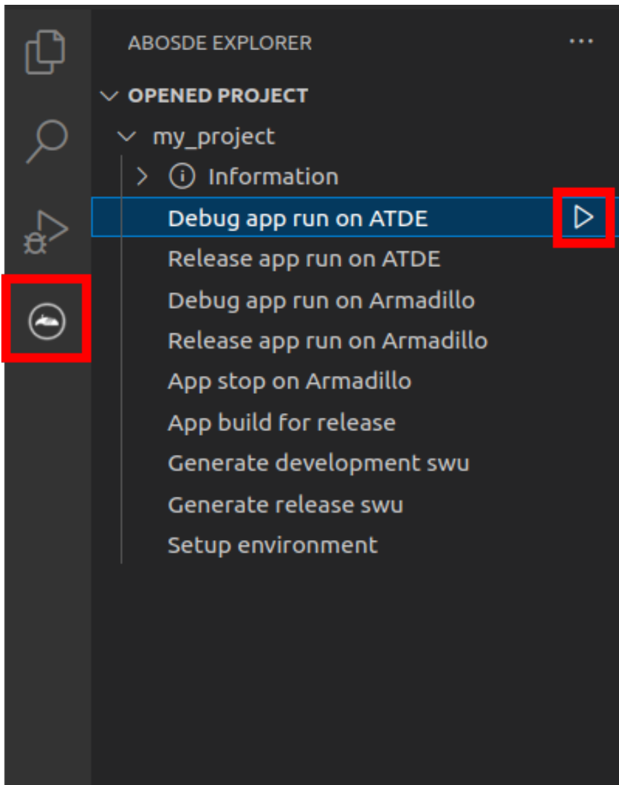
図 3.155 ATDE 上で Debug モードでビルドしたアプリケーションを実行する
