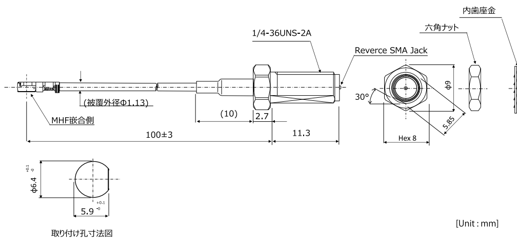
図 6.245 無線 LAN/BT 用アンテナケーブル形状図
