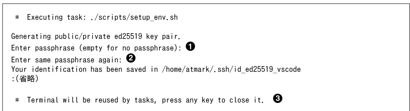
図 3.210 SSH 用の鍵を生成する
