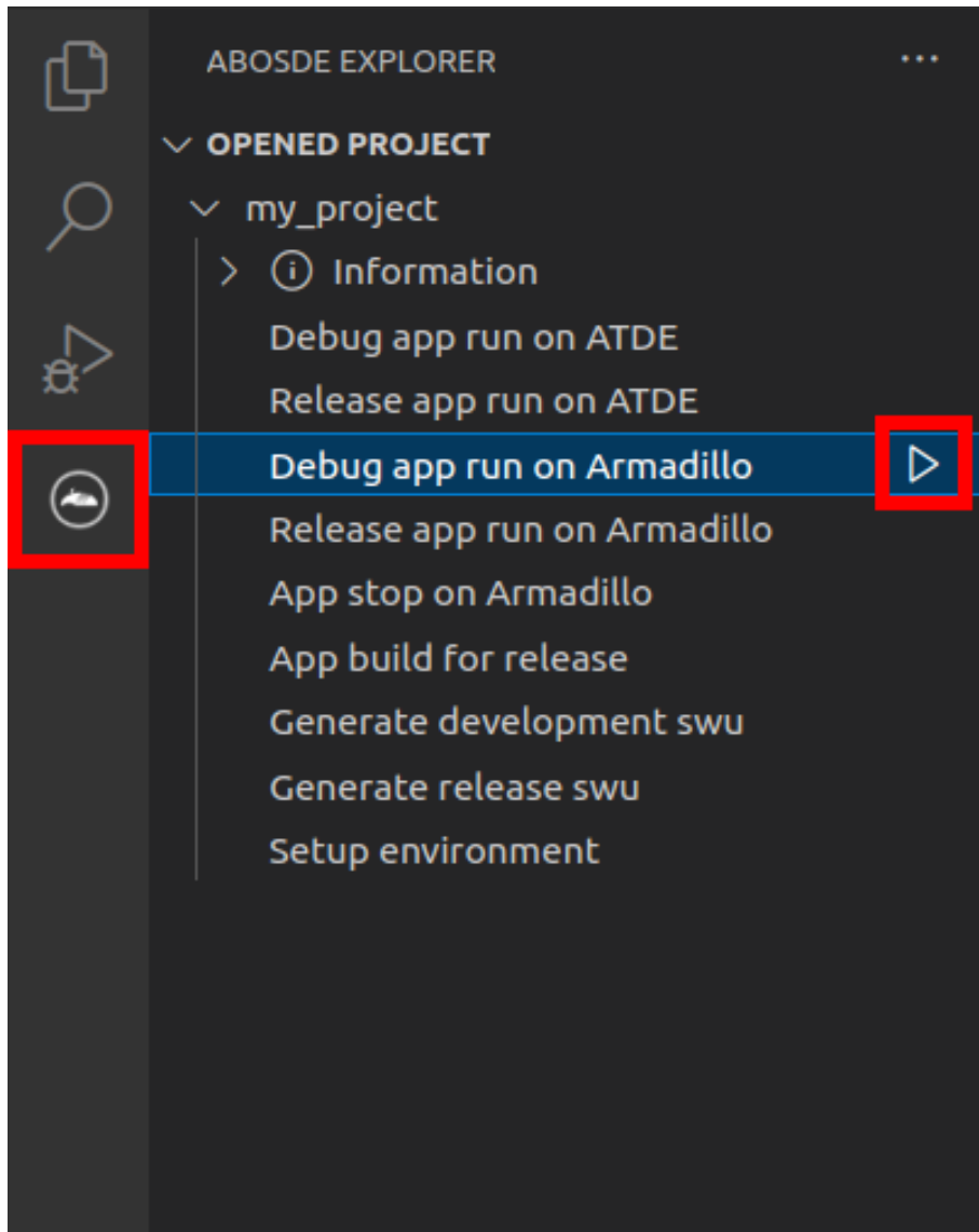
図 3.165 Armadillo 上で Debug モードでビルドしたアプリケーションを実行する
