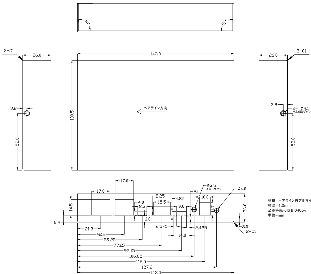
図 6.238 WLAN モデル ケース(上)形状図
