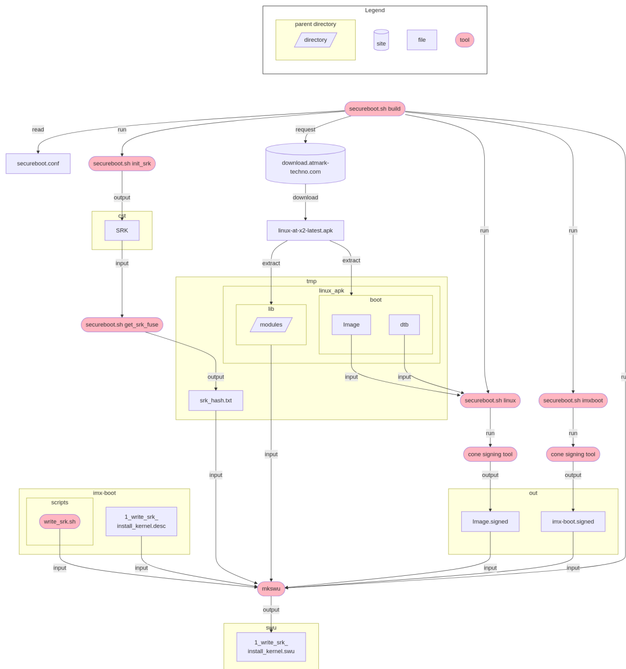
図 3.7 1_write_sr_k_install_kernel.swu を生成するまでの流れ
