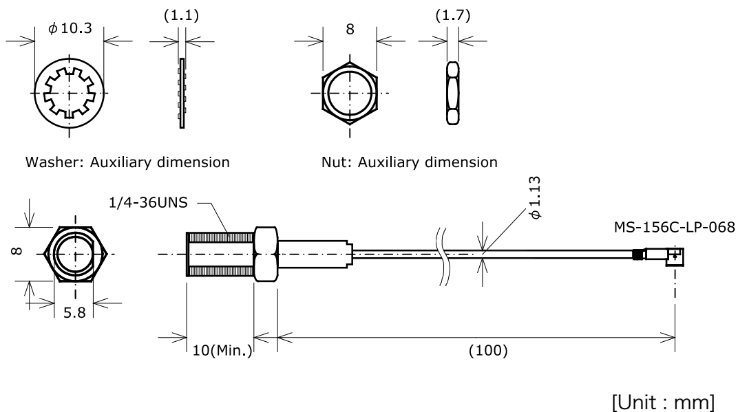
図 A.2 アンテナケーブル部の外形寸法図
