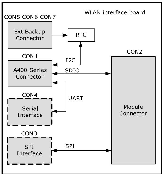
図 C.1 WLAN インターフェースボードのブロック図
