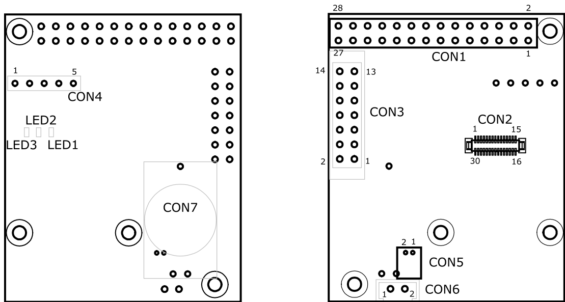
図 C.2 WLAN インターフェースボードのインターフェース配置
