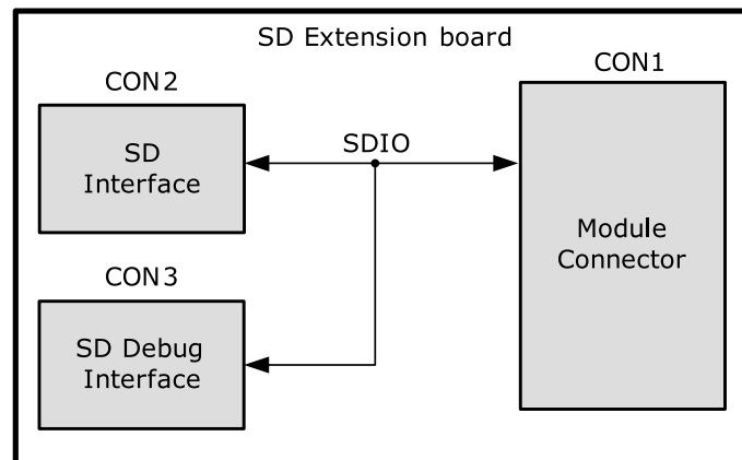
図 D.1 SD 変換ボードのブロック図
