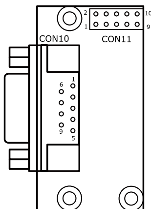
図 C.4 RS232C レベル変換ボードのインターフェース配置
