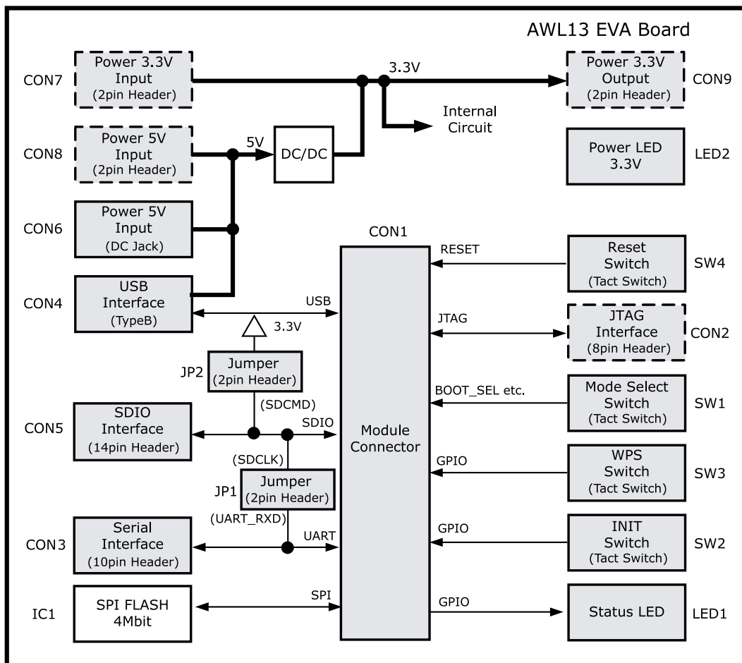
図 C.1 AWL13 評価ボード 本体のブロック図
