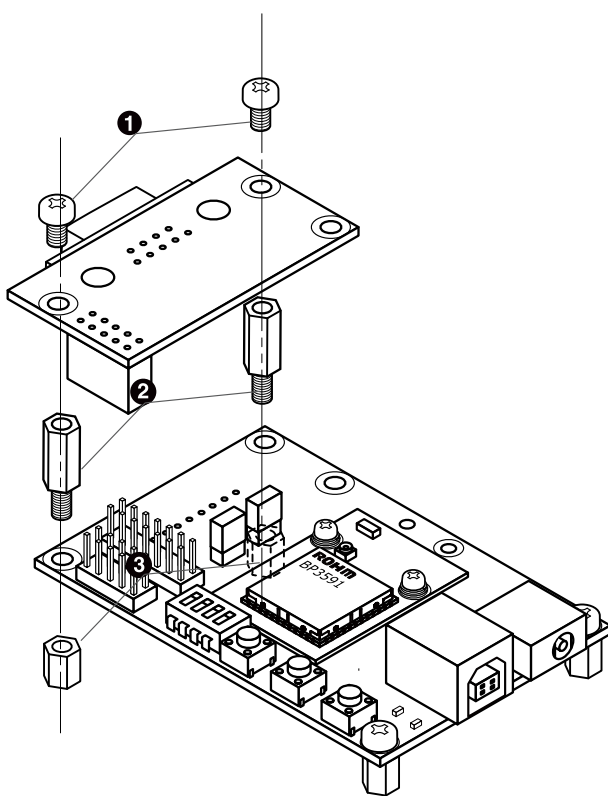
図 C.10 AWL13 評価ボードと RS232C レベル変換ボードの組み立て
