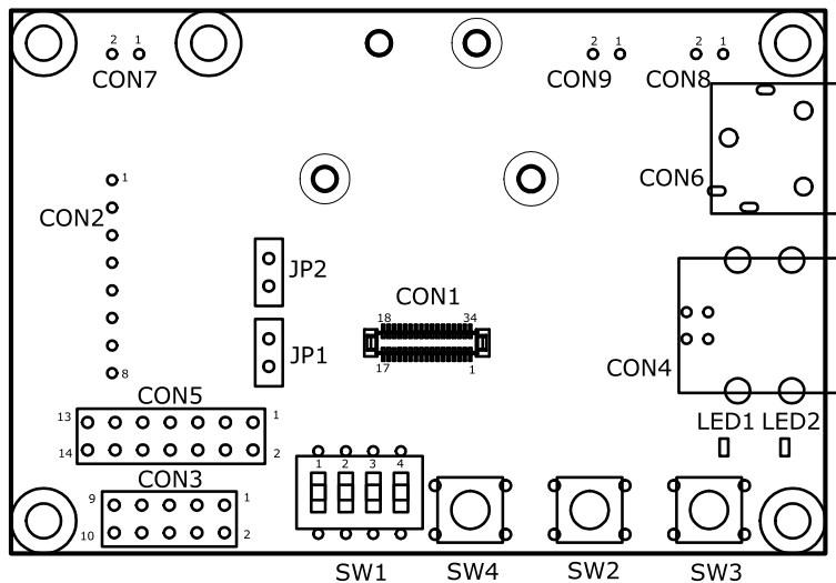
図 C.3 AWL13 評価ボード 本体のインターフェース配置
