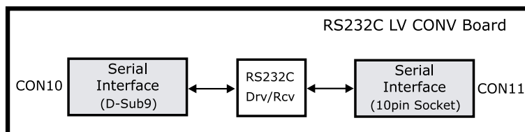
図 C.2 RS232C レベル変換ボードのブロック図
