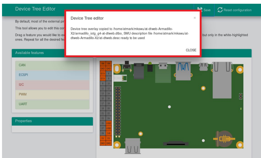
図 9.187 dtbo/desc の生成完了
