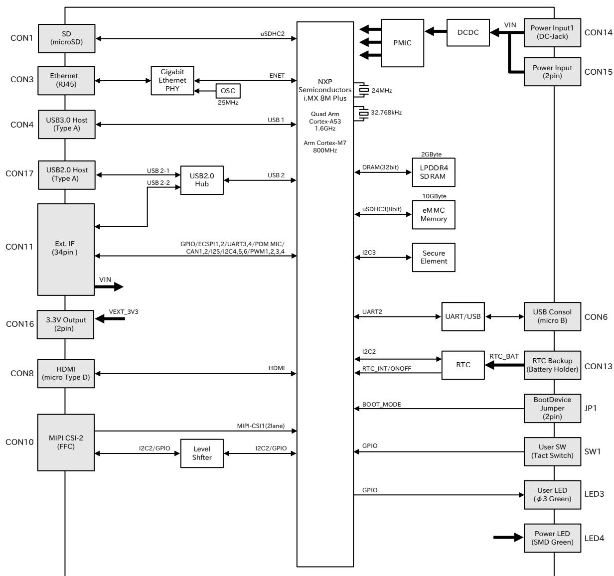
図 3.9 ブロック図
