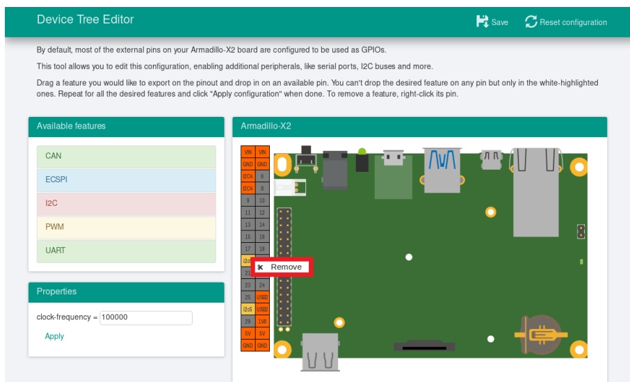
図 9.185 I2C5(SCL/SDA) の削除
