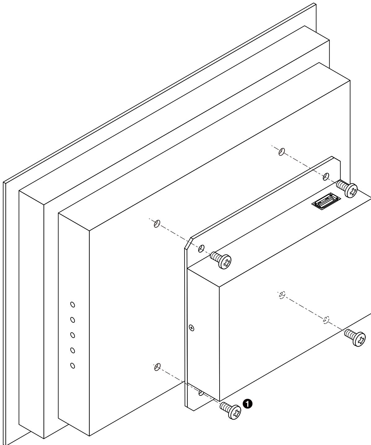
図 13.29 モニターに VESA 規格固定用プレートを取り付け
