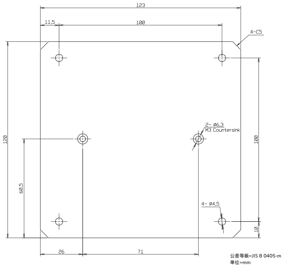
図 6.193 Armadillo-X2、G4 ケースモデル VESA 規格固定用プレート形状図
