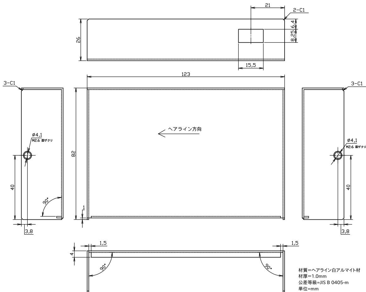
図 6.187 ケース(上)形状図
