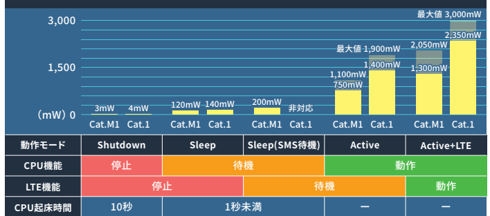
動作モードと消費電力 ※参考値
