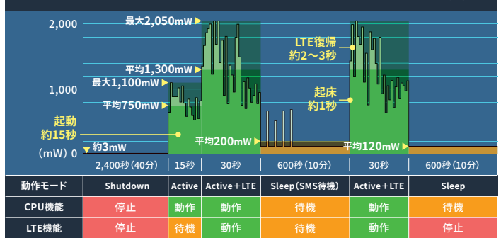
間欠動作時間の例と消費電力 ※Cat.M1モデルの参考値
